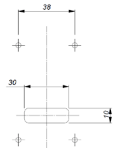
Panel Cutout : 12 way
